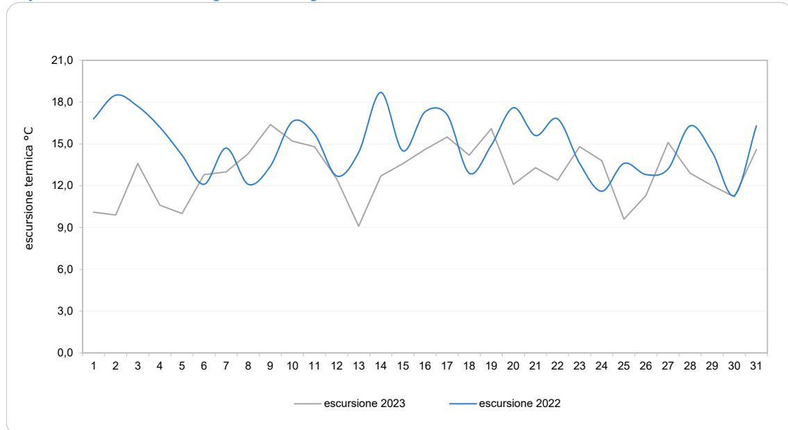
Grafico 2 – Escursione termica giornaliera. Luglio 2023 e 2022.
