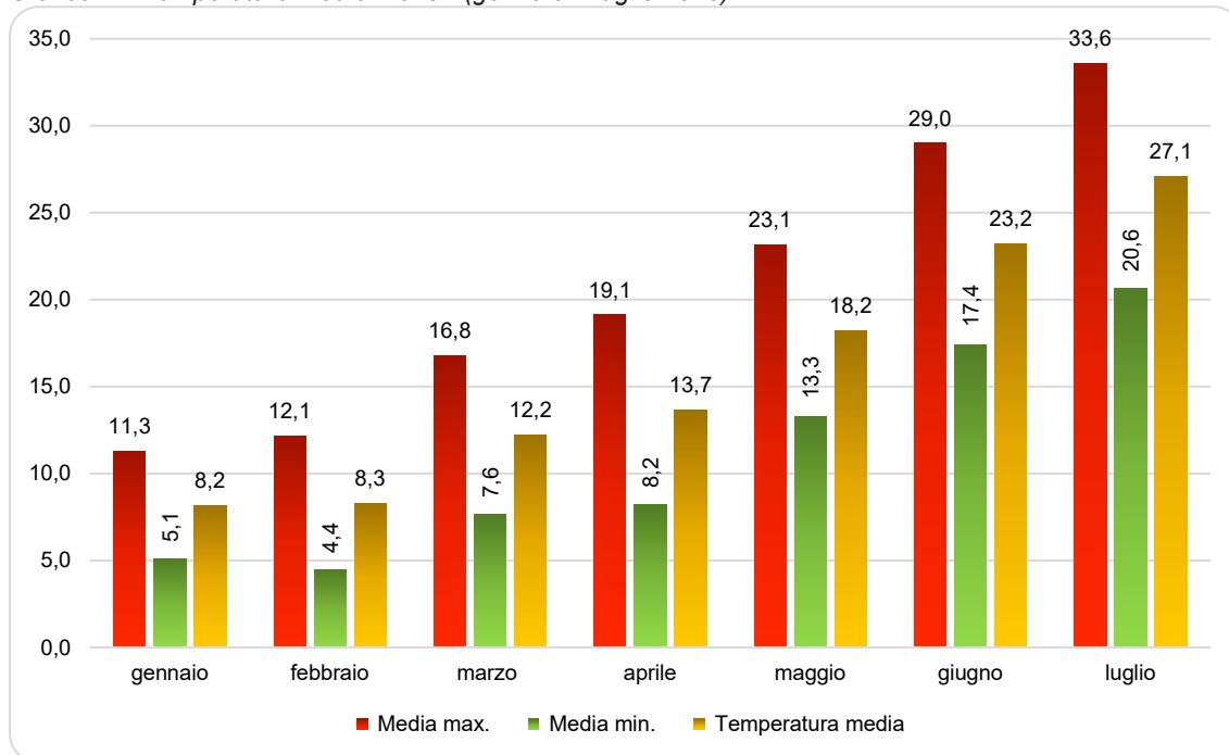
Grafico 4 – Temperature medie mensili (gennaio – luglio 2023).
