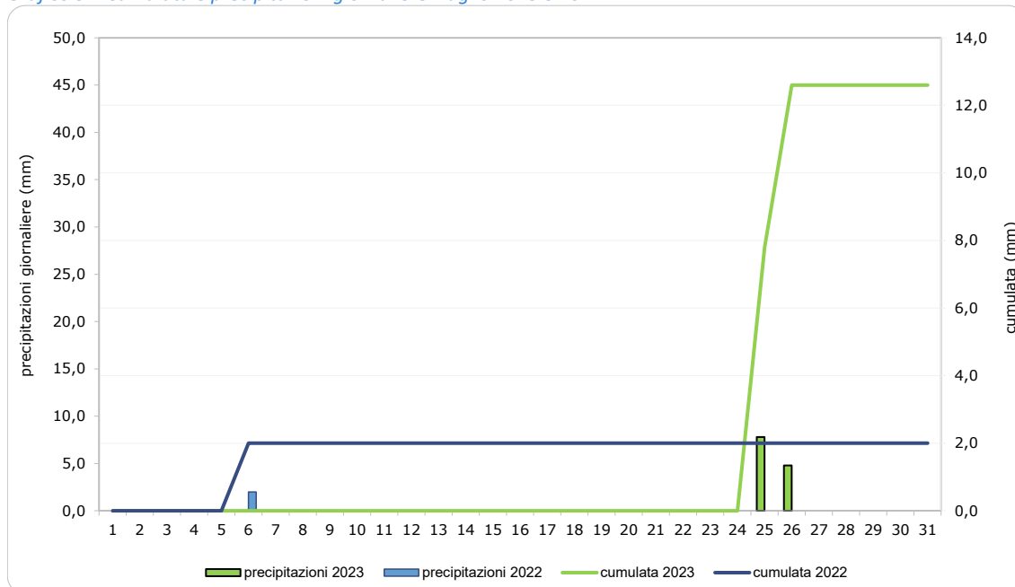
Grafico 5 – Cumulata e precipitazioni giornaliere. Luglio 2023 e 2022.
