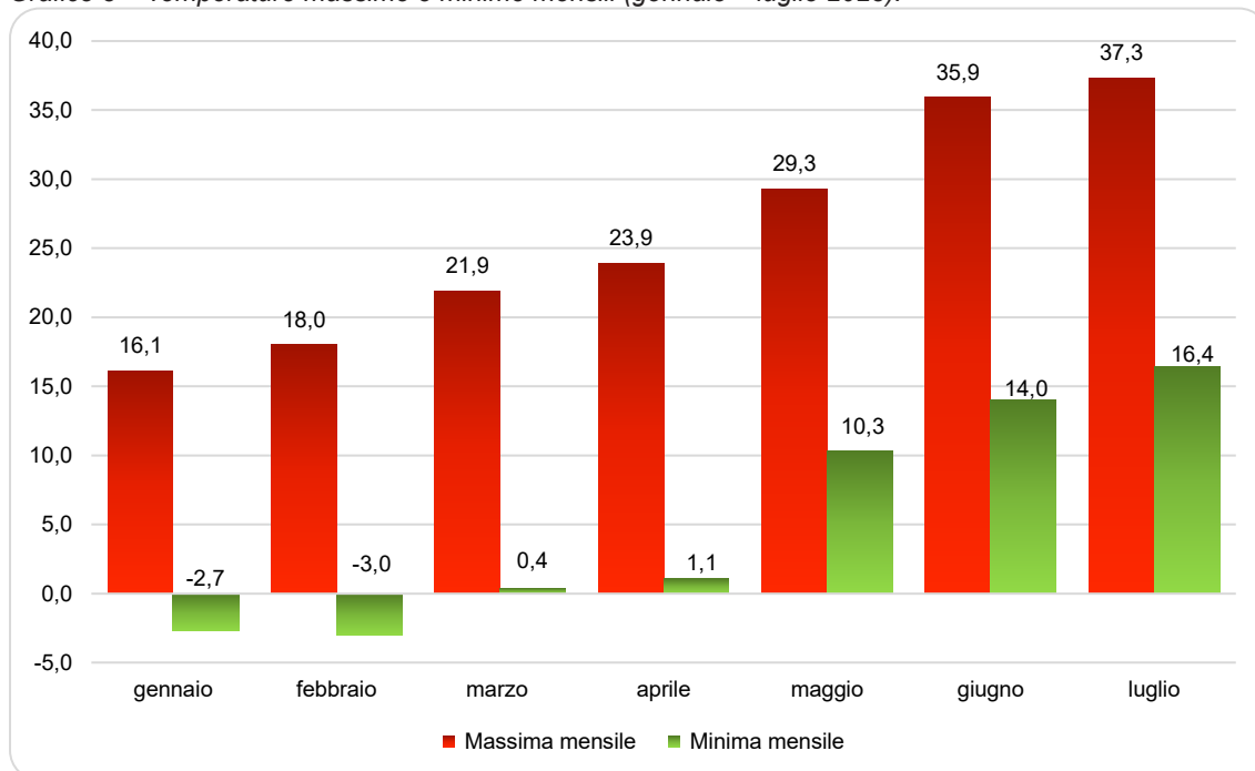
Grafico 3 – Temperature massime e minime mensili (gennaio – luglio 2023).
