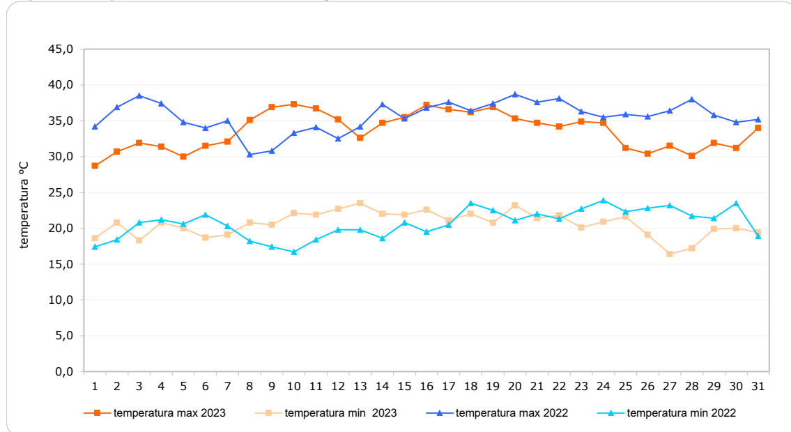
Grafico 1 – Temperature massime e minime. Luglio 2023 e 2022
